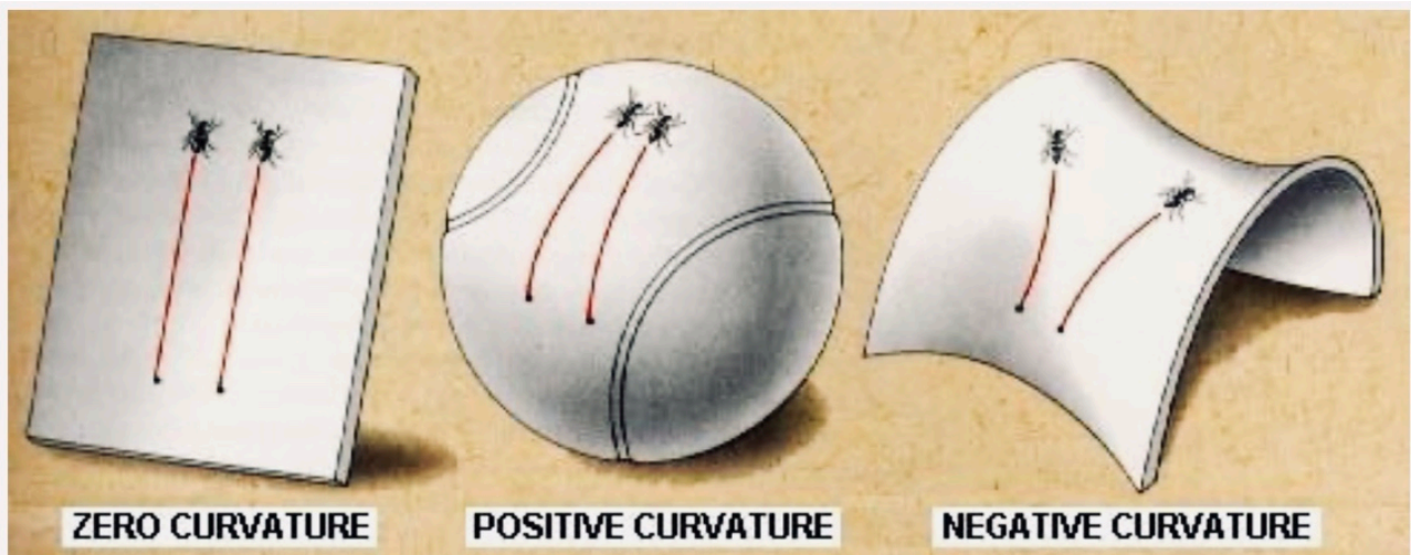
شکل 30: نماذج فریدمان
