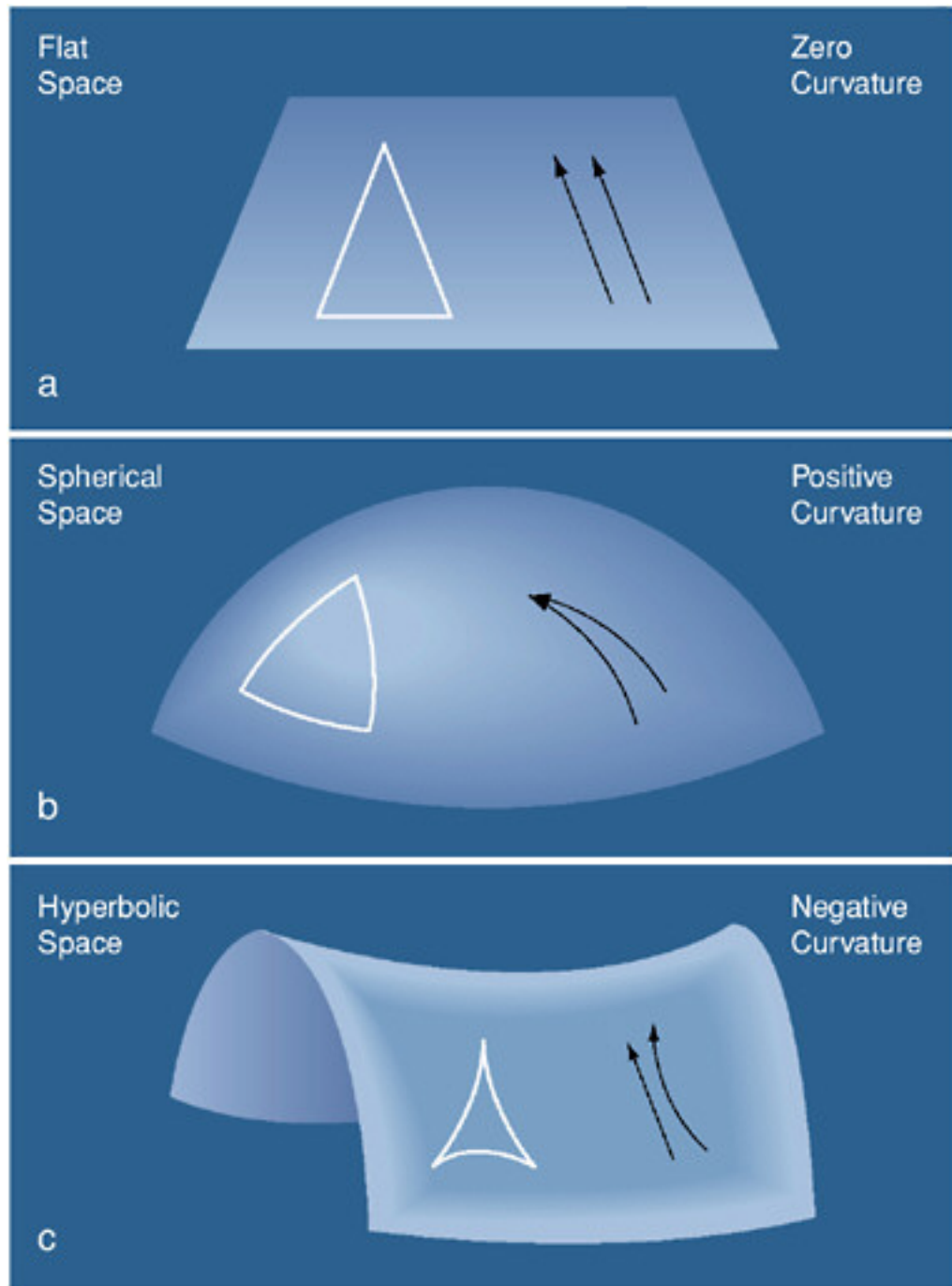
شکل 24: نماذج فریدمان (1)
