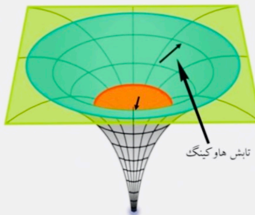
شکل ۲۳: تشریح تابش هاوکینگ، چگونگی و مکان پیدایش آن
